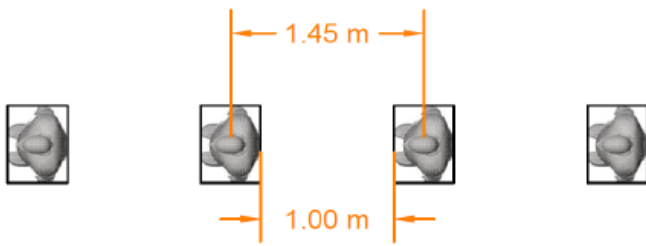
Abb. 2: einfache Warteschlange
