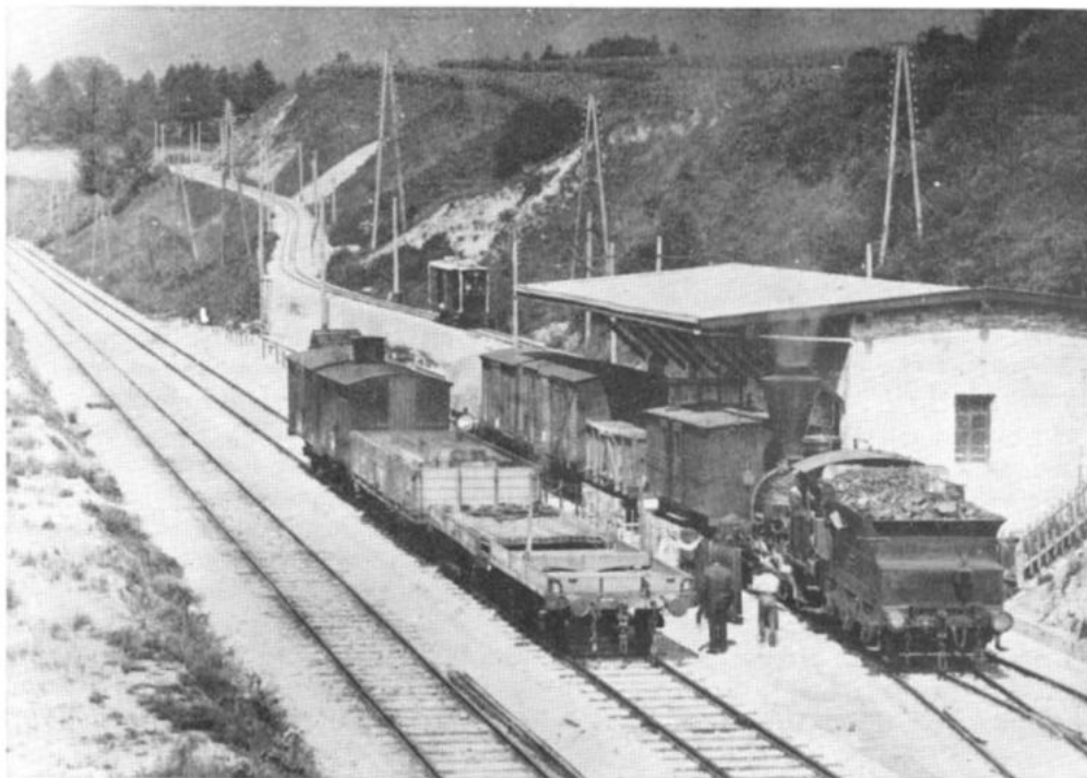
Die Verladerrampe an der Unterinntaler Staatsbahn mit der „Talstation“, dem kleinen Triebwagen und einem Stück Bahntrasse der schmalspurigen Schleppbahn der „Rauch-Mühle“. Im Jahre 1900 eröffnet, war dies die erste mit elektrischem Strom betriebene Bahnanlage Tirols (aufgelassen 1919).
